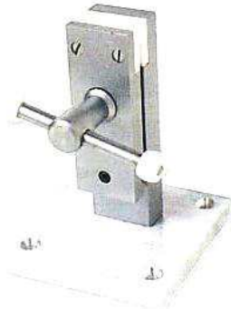
ET-107 ÉTAU en acier et socle aluminium avec mors nylon - Ouverture maximum : 12 mm Stainless steel VICE and aluminium base with nylon jaws - Maximum opening : 12 mm
